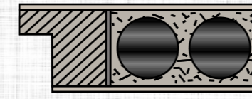
eckige Kante
